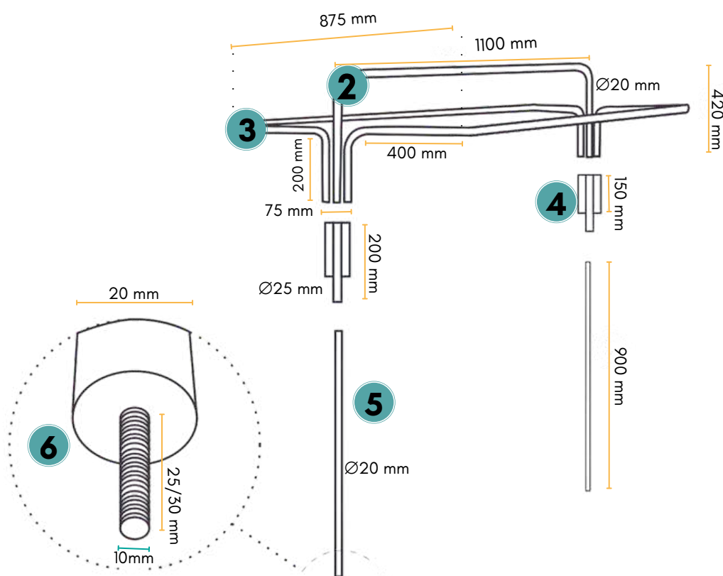
MEDIDAS DE PORTA-TOLDO
